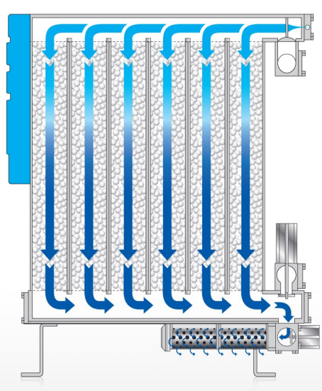
再生流程
