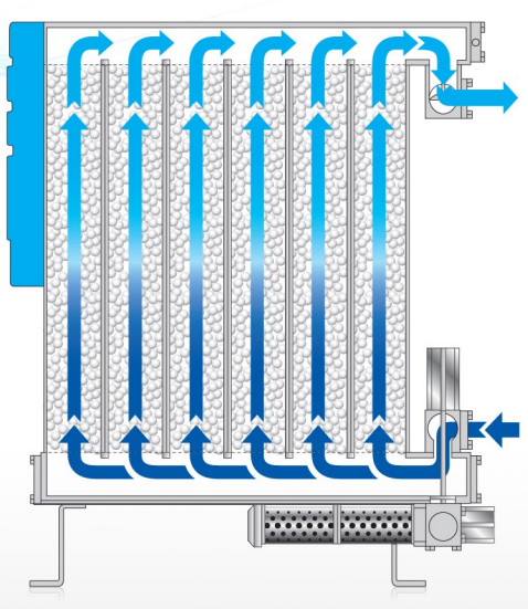
吸附流程
